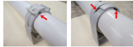
クリップの刃が一部噛み合っていない状態
