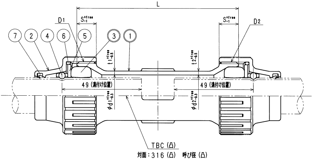
寸法表
