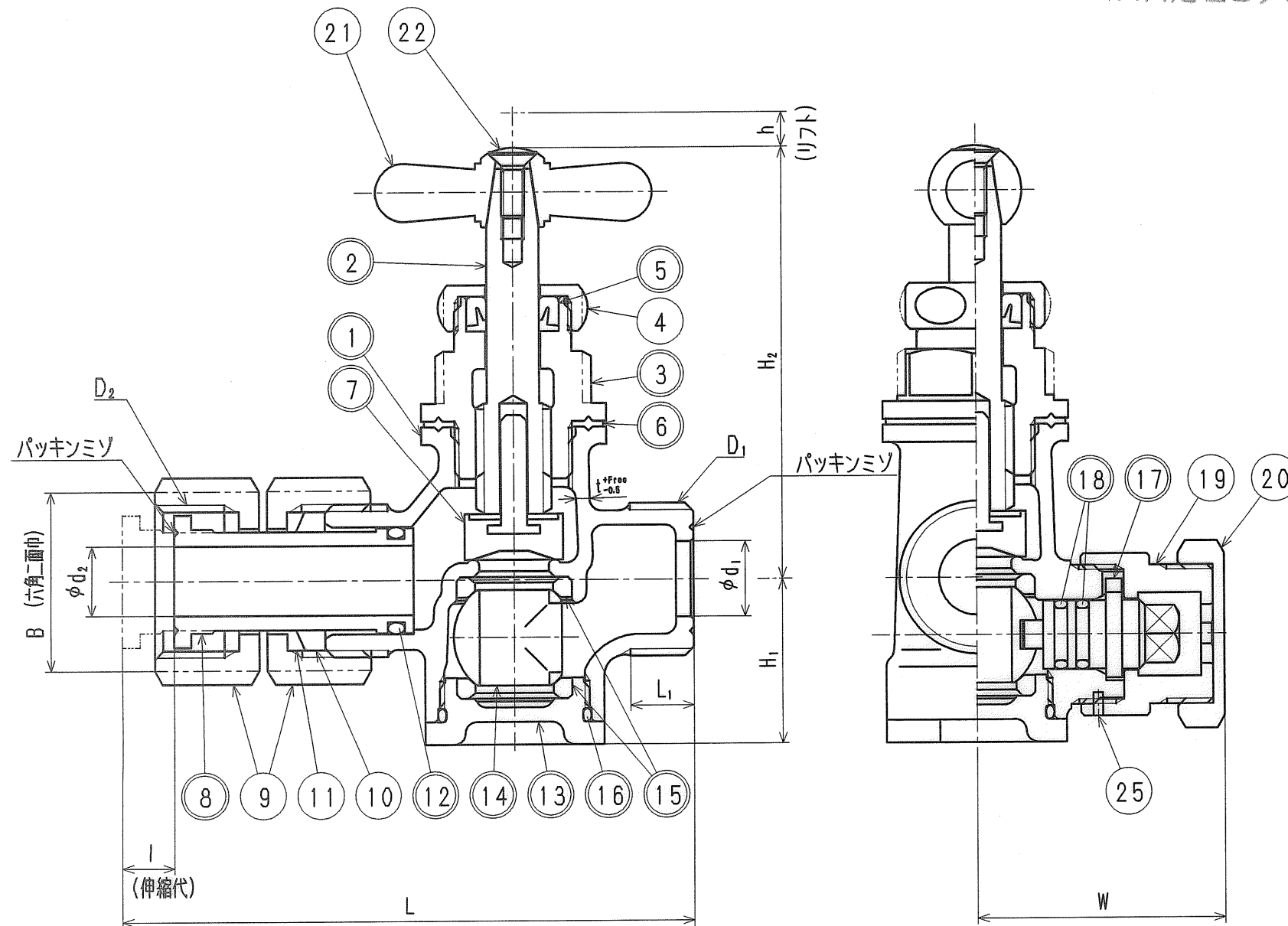
寸法表
