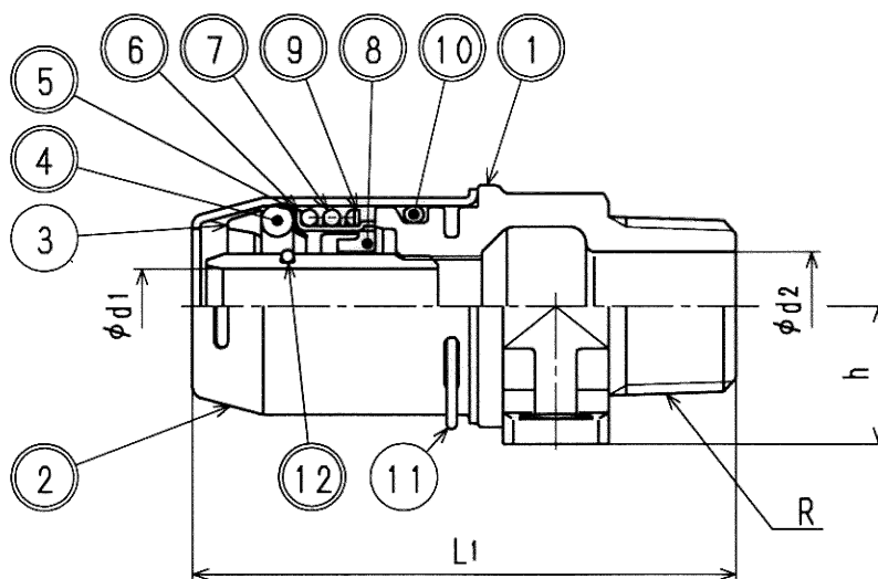
寸法表
