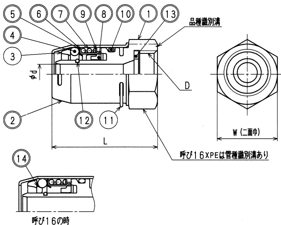
寸法表
