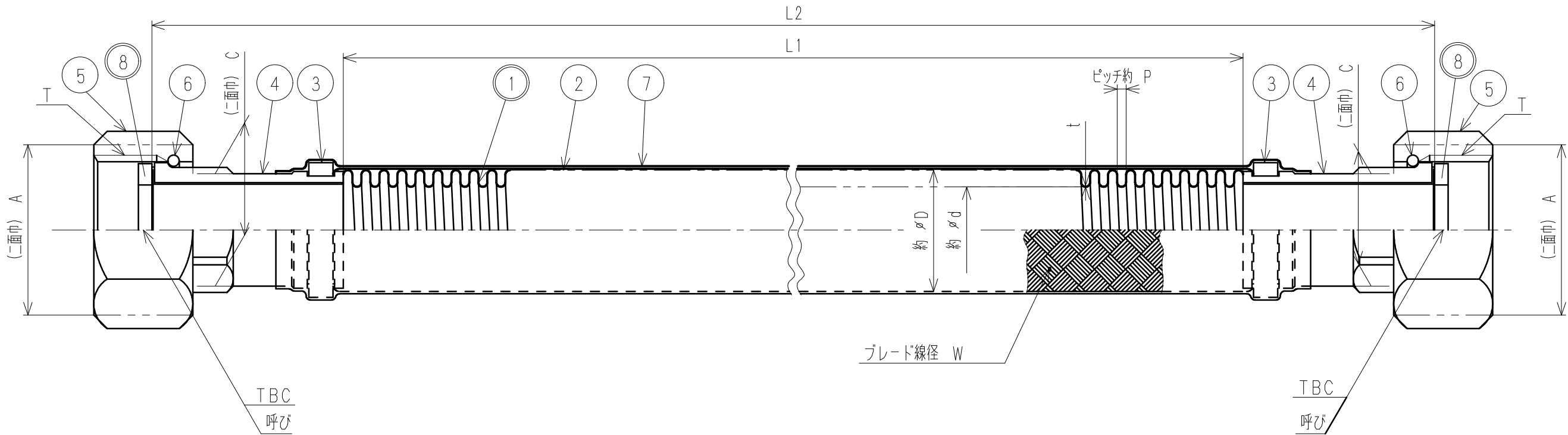
寸法表
